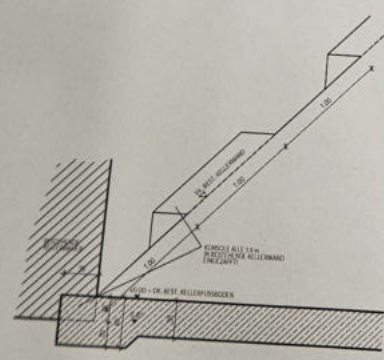
SCHNITT 1-1 FUNDIERUNGSVERSTÄRKUNG M 1:20
